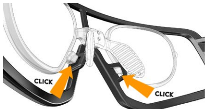
4 premere per agganciare il clip push to assemble the clip
